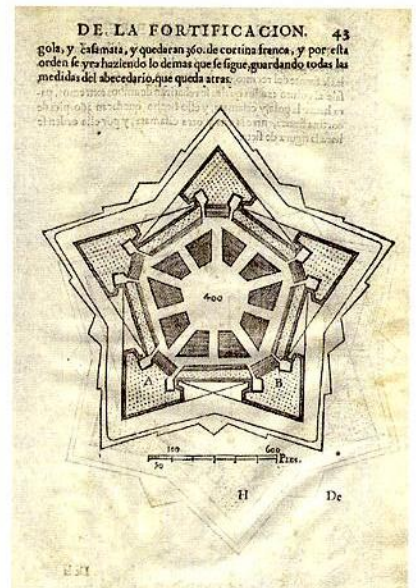
Teoría y práctica de fortificación. Christoval de Rojas, 1598.
